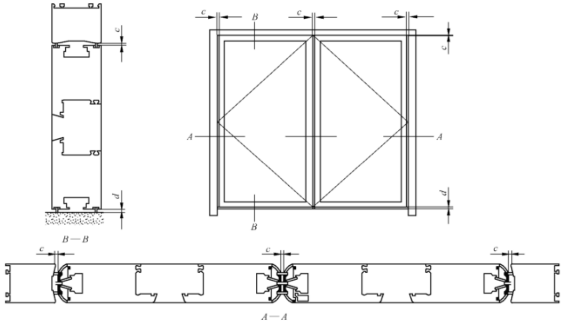
图 5 推拉门
